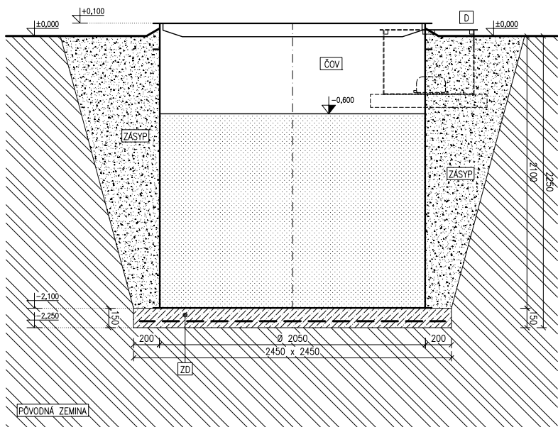
Разрез
